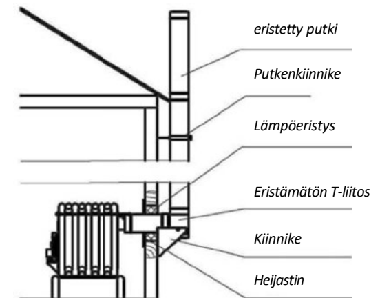
Kuva 6. Hormin asennus seinän läpi
