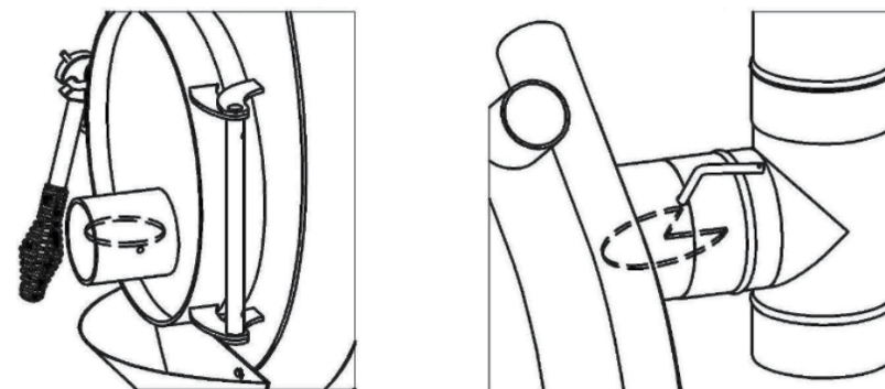
Kuva 11. Peltien asento lämmitysuunia sytytettäessä ja puita pesään lisättäessä (intensiivinen lämmitys)
