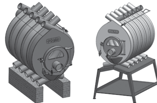
Kuva 2. Lämmitysuunin asennusvaihtoehdot
