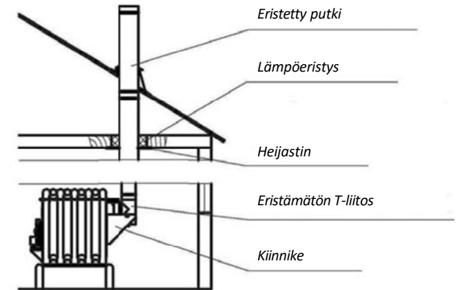
Kuva 5. Hormin asentaminen katon läpi
