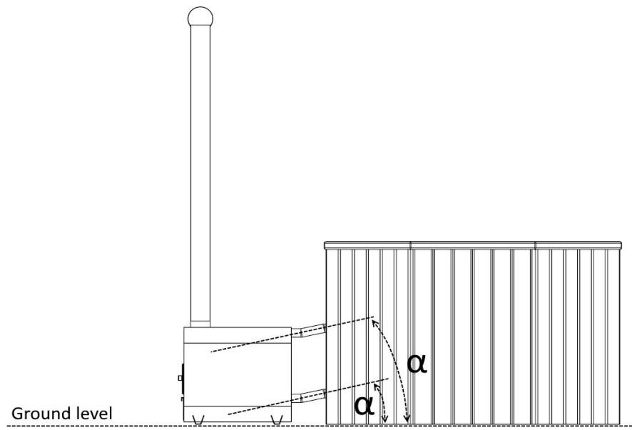
Kuva 3. Joustavien letkujen oikea asento ulkokamiinan yhdistämisessä kylpytynnyriin
