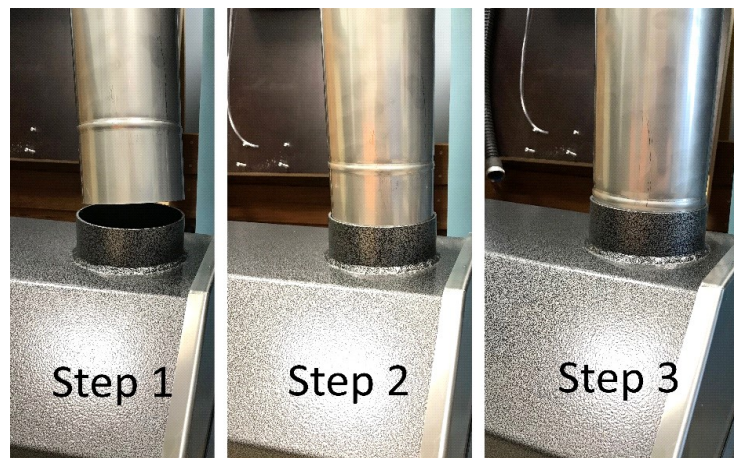
Kuva 7. Savupiipun asennus
